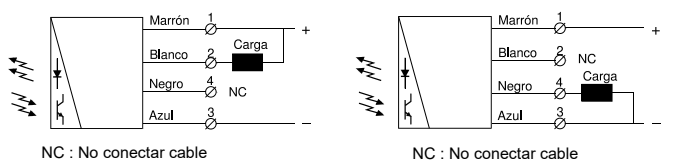
SPP 2603 / SPP 2605 Carga NPN
