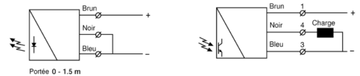
SMT 3000 Courte portée / SMR 32XX / SMR 33XX Sortie transistor PNP
