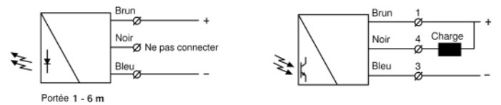
SMT 3000 Longue portée / SMR 30XX / SMR 31XX Sortie transistor NPN
