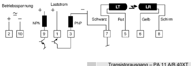
Transistorausgang - PA 11 A/B 40XT
