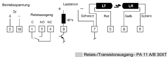
Relais-/Transistorausgang - PA 11 A/B 30XT
