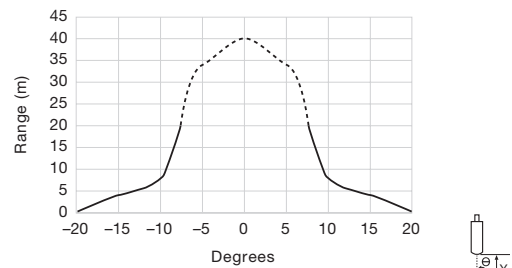
SMR 9x20
