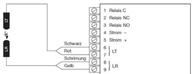
Relais-Ausgang
