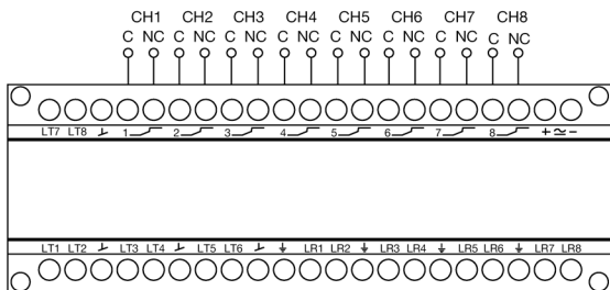
MPA 81 A/C 50X 8 sorties relais individuel
