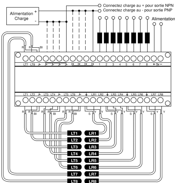
MPA 81 A/C 60X 8 sorties transistor individuel
