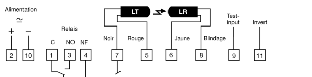
Sortie relais – PA 01 X 51X
