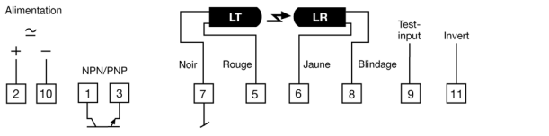
Sortie transistor – PA 01 X 61X
